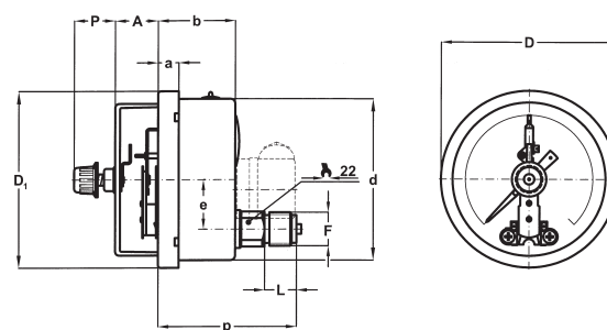
D - ЗАДНЕЕ ПРИСОЕДИНЕНИЕ
